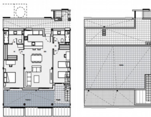
Plano
